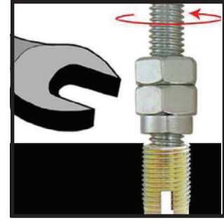
4. Takma Aparatını Ters Yönde Çıkartma İşlemi
