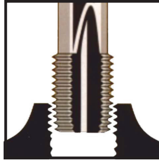
2. İşlem Kılavuz Çekme
