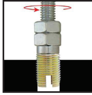
3. İşlem Vida Yönünde İnsört Yerleştirme
